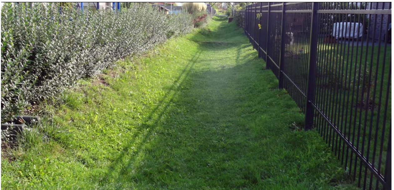
Gemeinsame Versickerungsmulde zwischen Grundstücken
